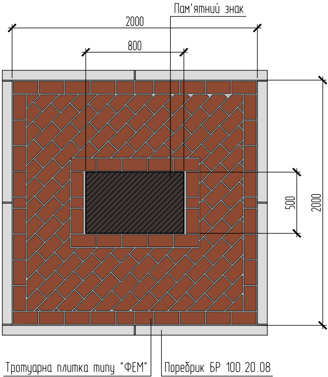
План майданчика М 1:30
